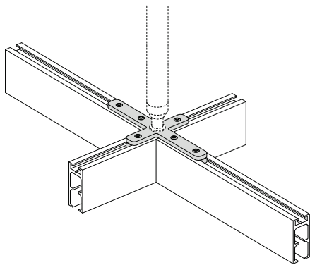
Kreuzverbinder
