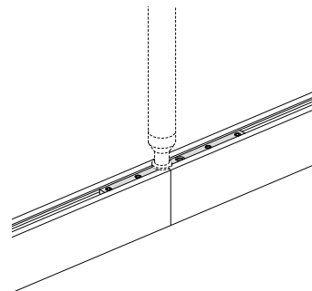
Stoßverbinder
