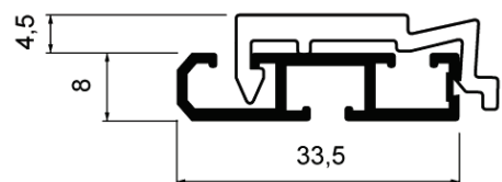
APS 1/2 1/2-läufig weiß lackiert silber lackiert highline titan
