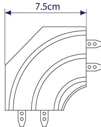
IAPS 2/3 für APS 2/3 3-läufig weiß oder silber lackiert
