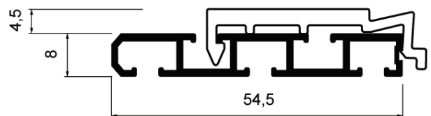
APS 2/3 2/3-läufig weiß lackiert silber lackiert highline titan
