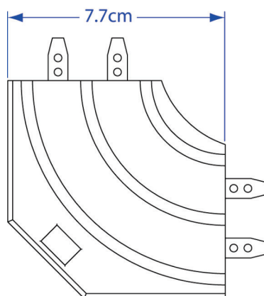
RAPS 2/3 für APS 2/3 3-läufig weiß oder silber lackiert
