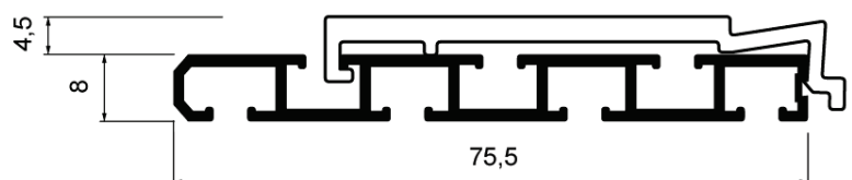
APS 2/3 2/3-läufig weiß lackiert silber lackiert highline titan
